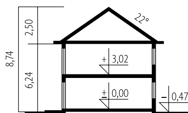
Schemat przekroju
