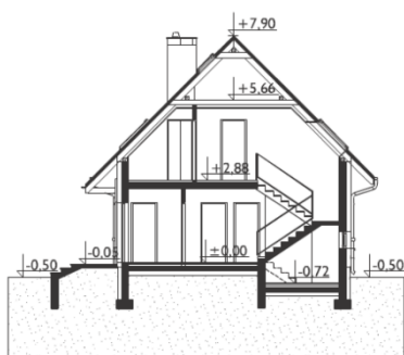
Schemat przekroju
