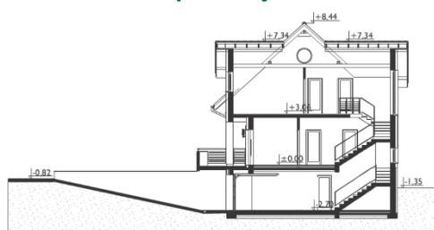
Schemat przekroju
