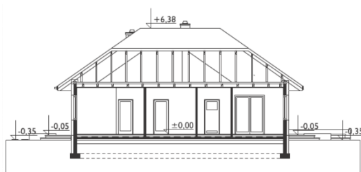
Schemat przekroju
