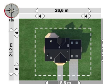
Usytuowanie na działce
