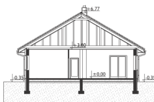
Schemat przekroju
